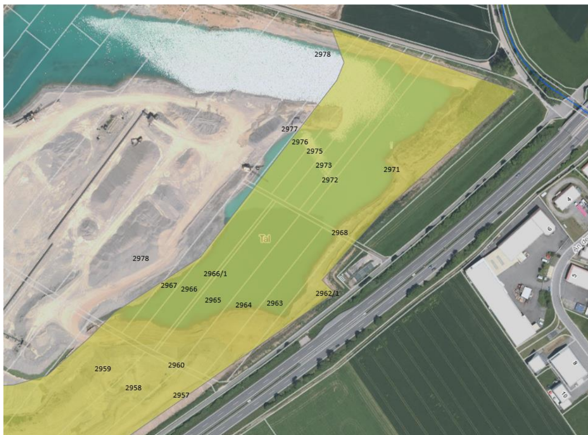
Abbildung 35: Flächen für den Oberbodenauftrag gem. ÖKVO (gelbe Flächen) – Detailplan 3
